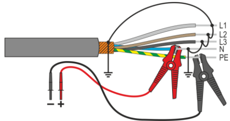
Abb. 3.2. Messung geschirmter Kabel
