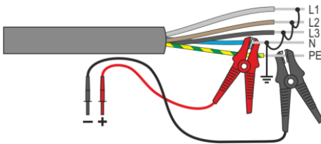
Abb. 3.1. Messung ungeschirmter Kabel
